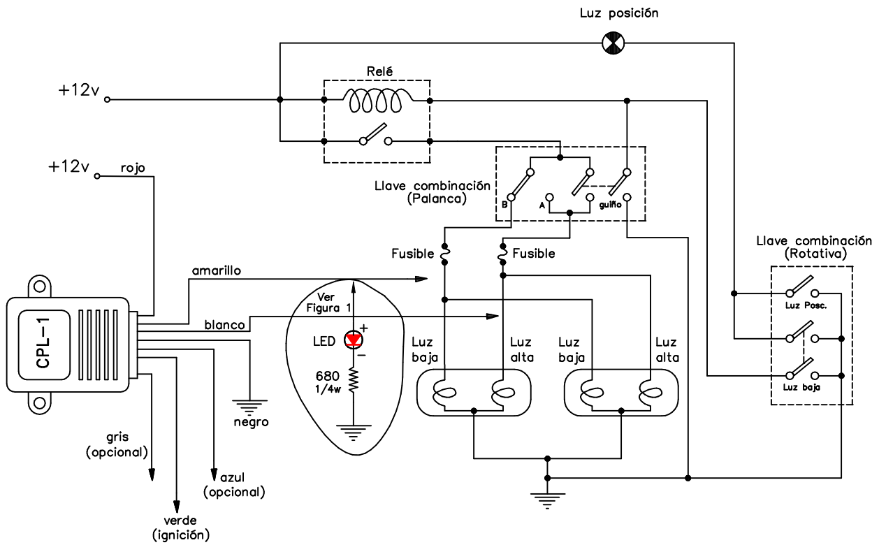
Diagrama Eléctrico
