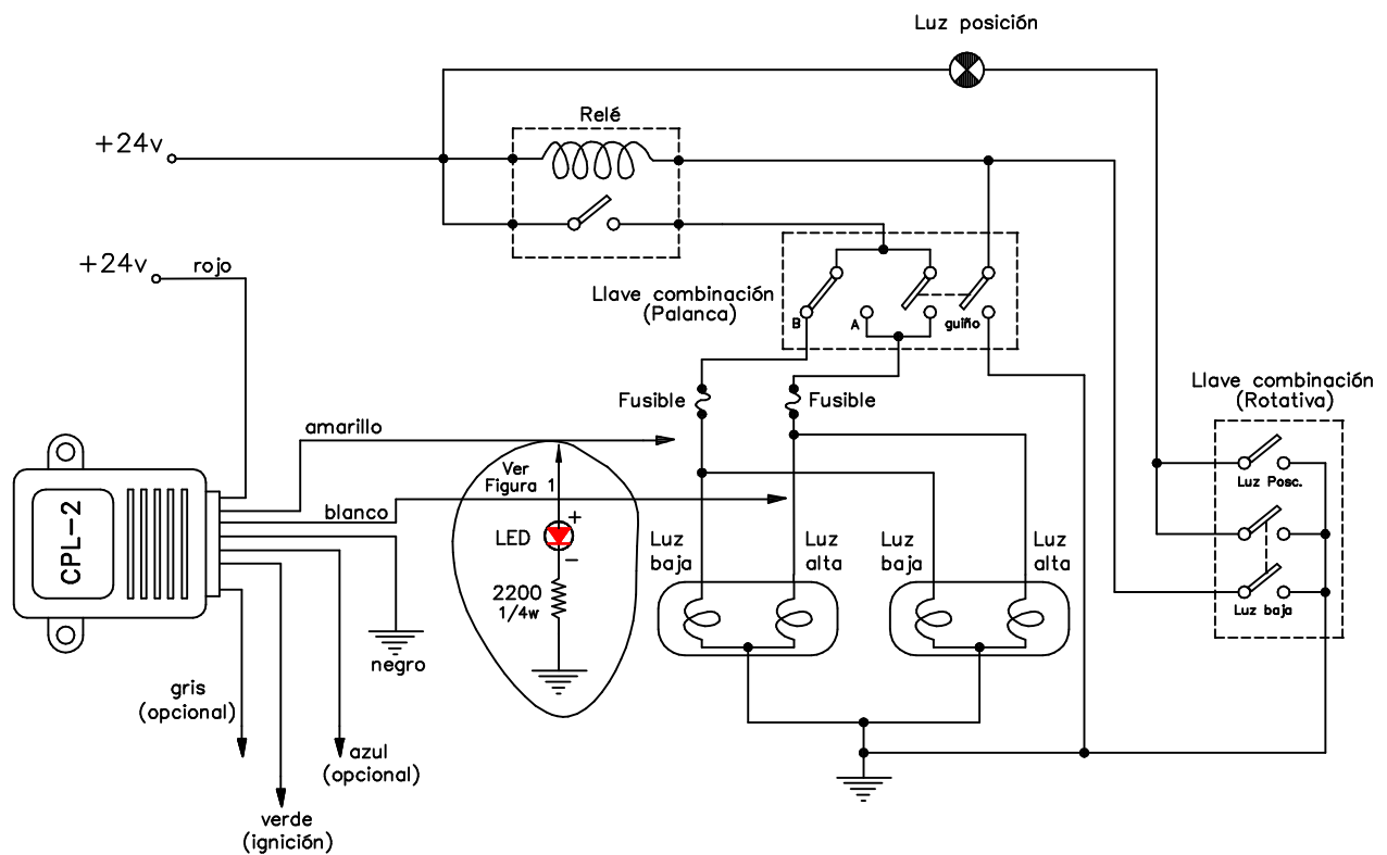
Diagrama Eléctrico
