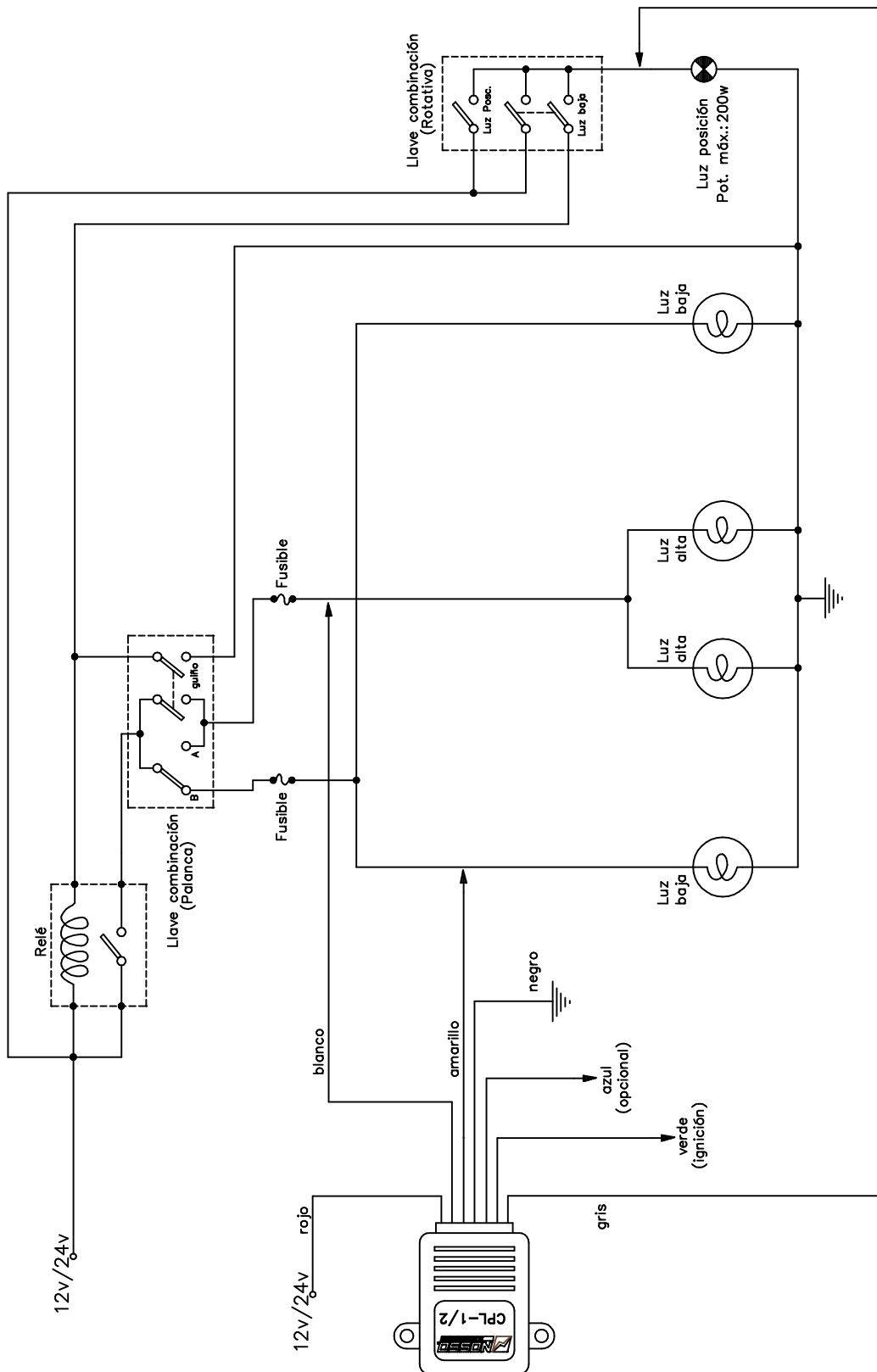
DIAGRAMA ILUSTRATIVO Lámparas Bajas separadas con terminal común a masa (Sistema EUROPEO-AMERICANO)
