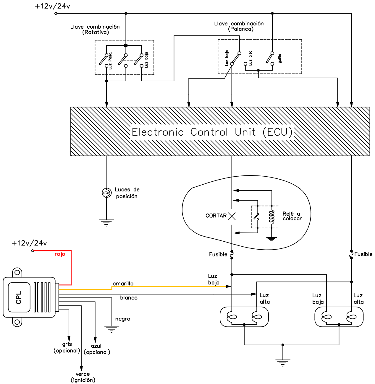
DIAGRAMA ILUSTRATIVO (Vehículos con ECU)
